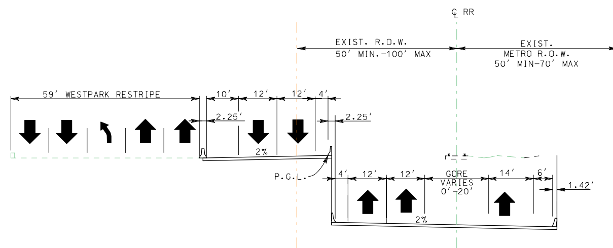
STA. 470+14 TO 476+00
