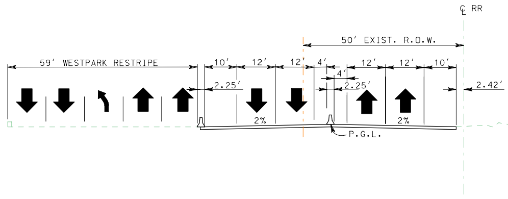
STA. 460+00
