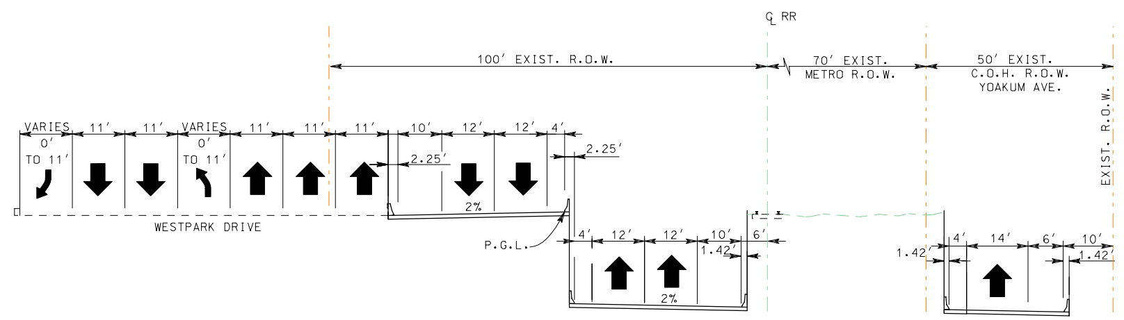
STA. 476+00 TO 482+00
