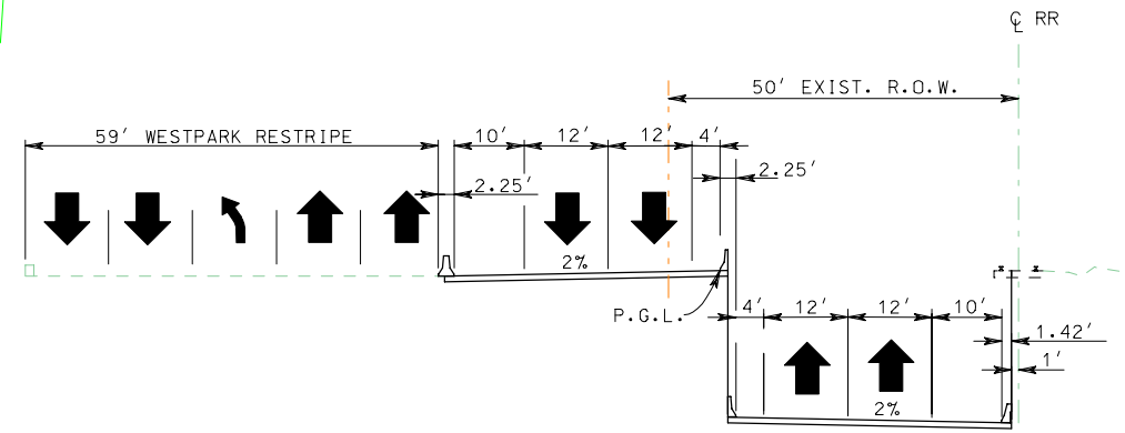
STA. 460+65 TO 470+14
