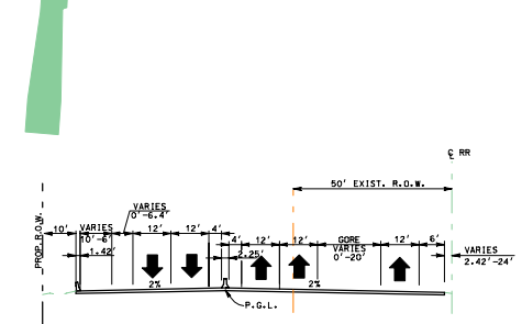
STA. 395+00 TO 413+50
