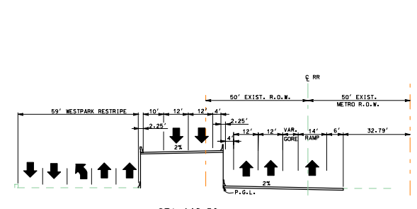
STA. 448+50
