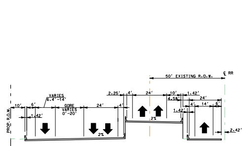
STA. 413+50 TO 423+00
