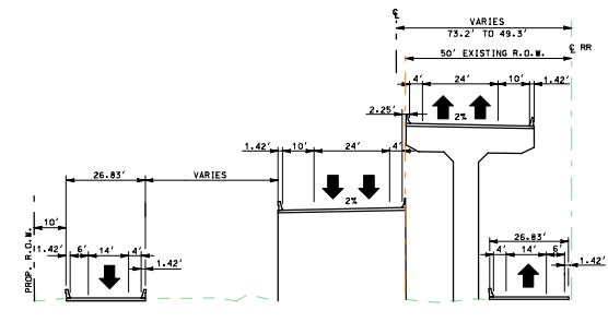
STA. 426+00 TO 433+00
