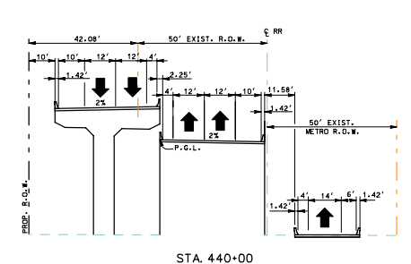
STA. 440+00
