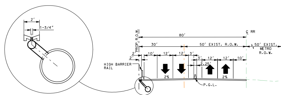
STA. 280+00 TO 310+00
