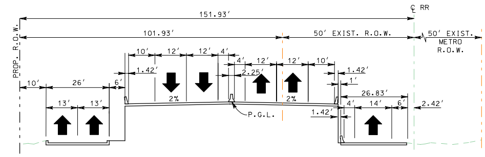
STA. 267+00
