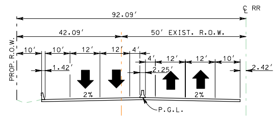
STA. 206+00 TO 212+00 STA. 239+00 TO 250+00
