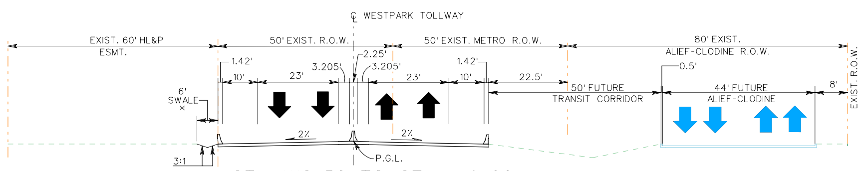
STA. 112+50 TO STA. 1119+00= STA. 119+00 TO STA. 150+00 (FUTURE TYPICAL SECTION)
